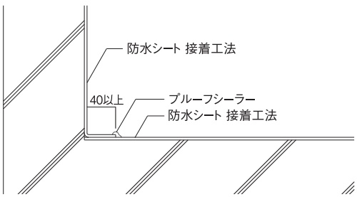
110仕様(RC下地の場合)
