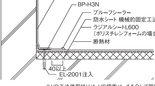
225、227仕様(US固定部)
