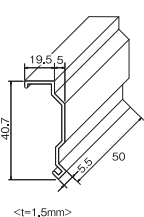
●K-11 ジョイナー
