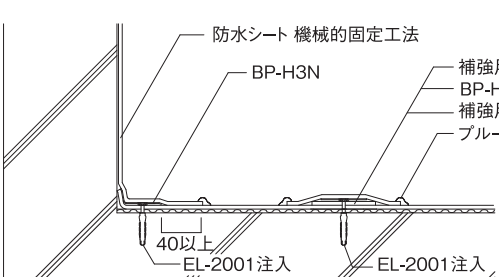
210US仕様(立上り機械的固定)
