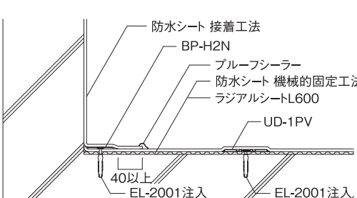
210UD仕様(立上り接着)
