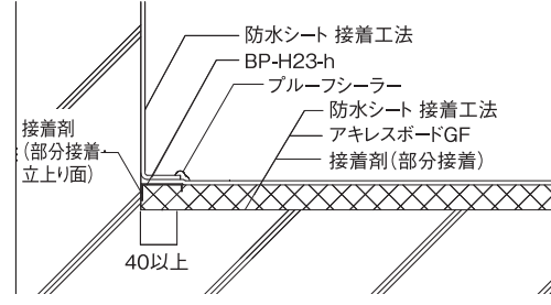
125、127仕様(RC下地の場合)
