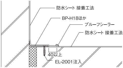
110仕様(ALC下地の場合)
