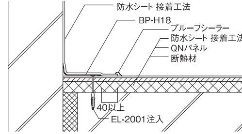
125、127仕様(ALC下地の場合)
