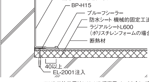
225、227仕様(UD固定部)
