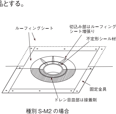
図 9.4.18 ルーフトレン回りの納まりの例
