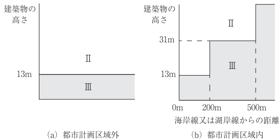
図1 地表面粗度区分II概略図
