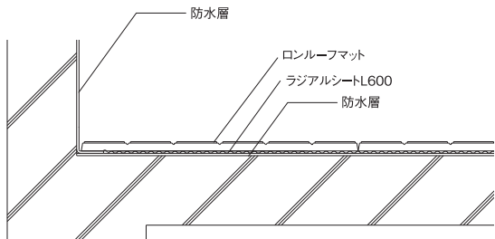
RM-1(RM-1C) 非断熱工法 断面
