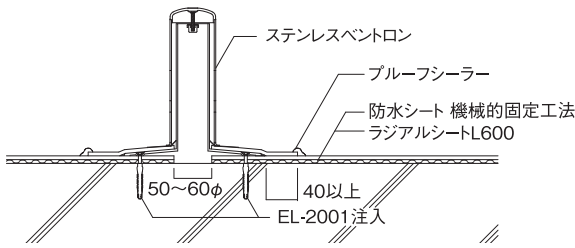
225、227仕様(ステンレスベントロン)
