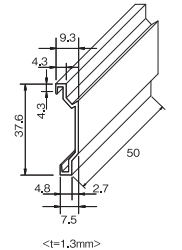
●K-8 ジョイナー
