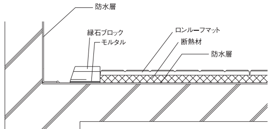
RM-2(RM-2C) 断熱工法 断面
