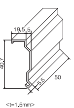
●K-11 ジョイナー
