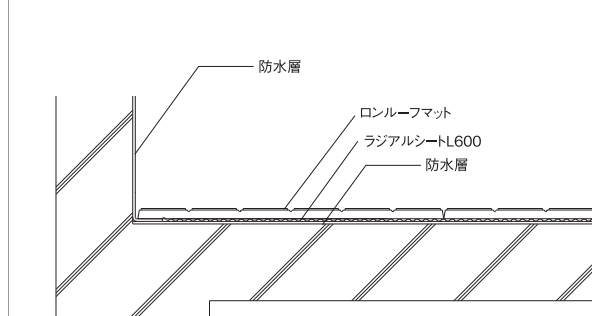
RM-1(RM-1C) 非断熱工法 断面
