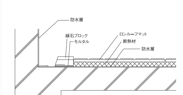
RM-2(RM-2C) 断熱工法 断面
