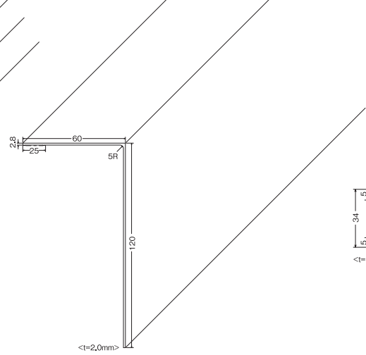
●K-11 ℓ=2000 <7穴>
