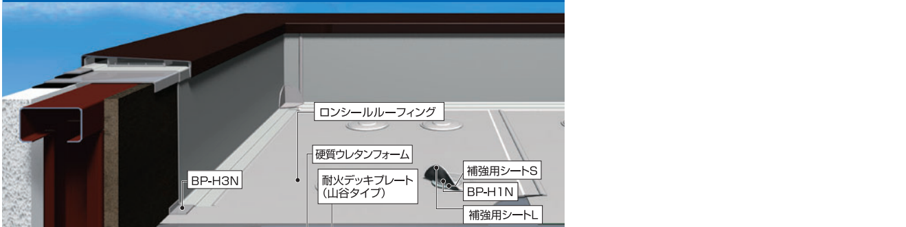
イメージ図 SD-S UD(225D UD)仕様の構造を表すイメージ図です。実際とは多少異なります。
