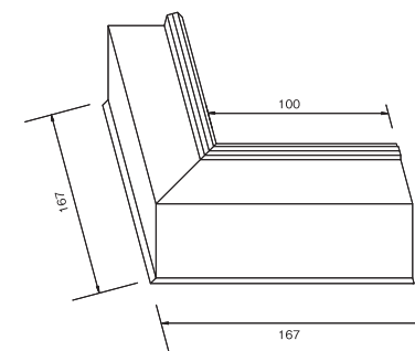
●K-10 出隅
