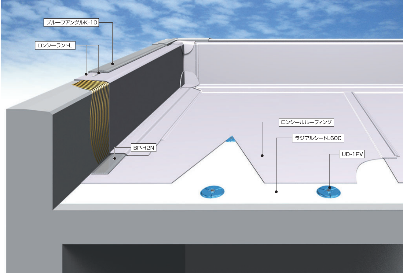
〈入隅鋼板 後付け〉
