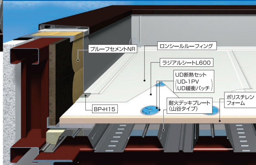
イメージ図 SD-S UD(225D UD)仕様の構造を表すイメージ図です。実際とは多少異なります。
