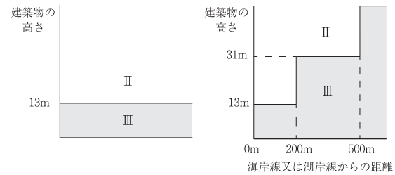
図1 地表面粗度区分II概略図
