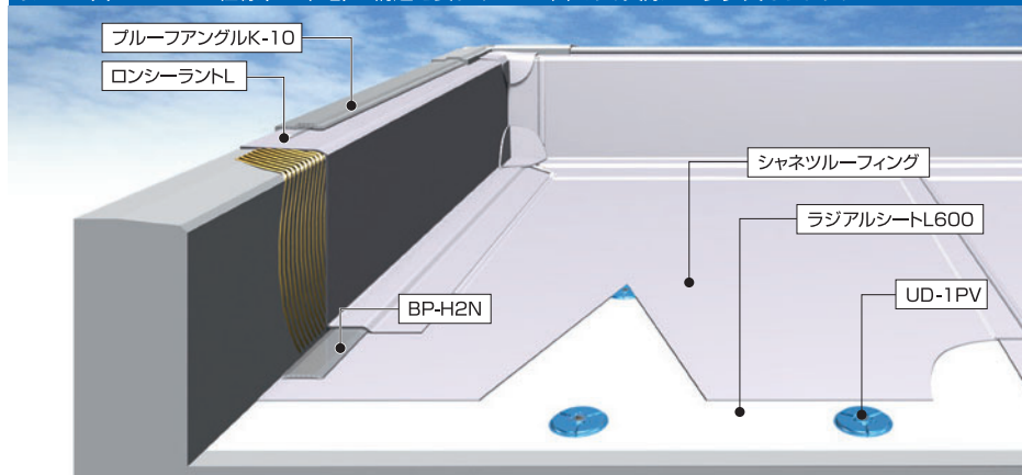
イメージ図 225 UD仕様(RC下地)の構造を表すイメージ図です。実際とは多少異なります。
