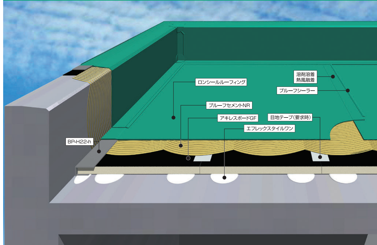
イメージ図 126仕様(RC下地)の構造を表すイメージ図です。実際とは多少異なります。
