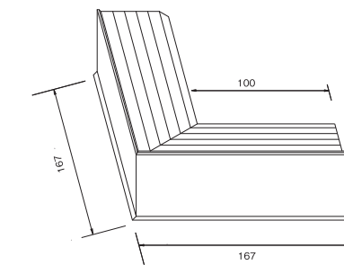
●K-13 出隅
