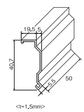
●K-11 ジョイナー
