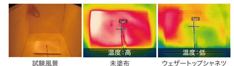
■ランプ照射試験(サーモグラフによる比較)
