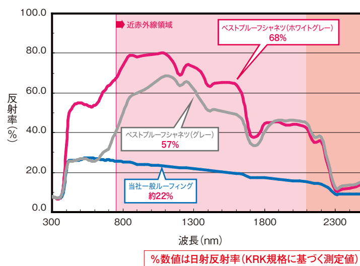
■図2 分光反射率グラフ(300nm～2500nm)
